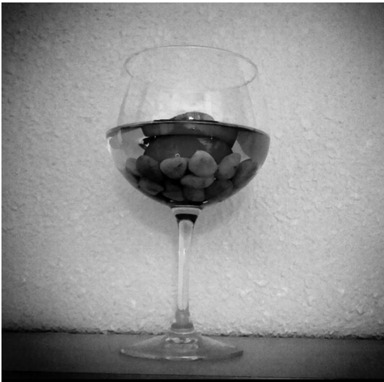
Equilibrio del H 2 O
